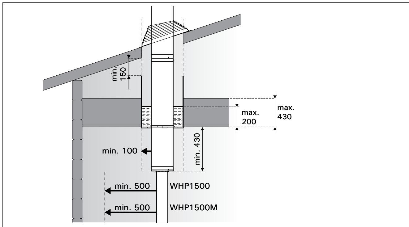
Рисунок 2. Безопасные расстояния (все размеры приведены в миллиметрах)
