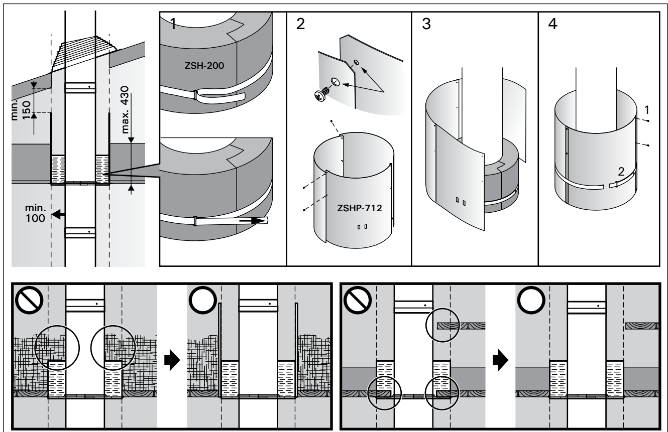
Kuva 3. Läpivienti (mitat millimetreinä) Bild 3. Genomföring (måtten i millimeter)
