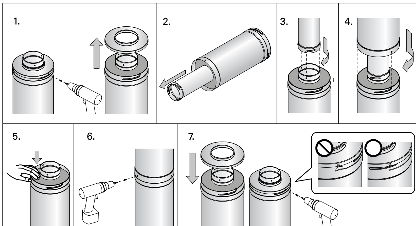
Рисунок 4. Соединение элементов дымохода между собой
